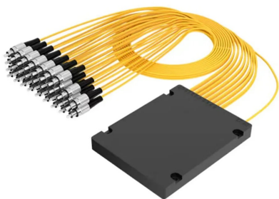
PLC en caja 1x8 · FC/UPC KG-FO-PLC-BOX-1X8-FCUPC Imagen de referencia de la serie
