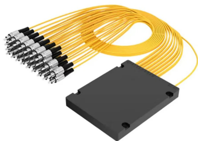
PLC en caja 1x16 · FC/UPC KG-FO-PLC-BOX-1X16-FCUPC Imagen de referencia de la serie
